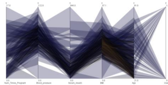
(d) Anonymization with k=4
